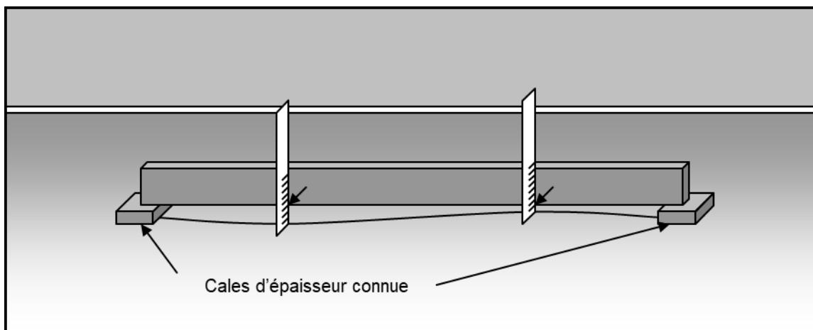
Figure 1 : Méthode de mesure des écarts de planéité
